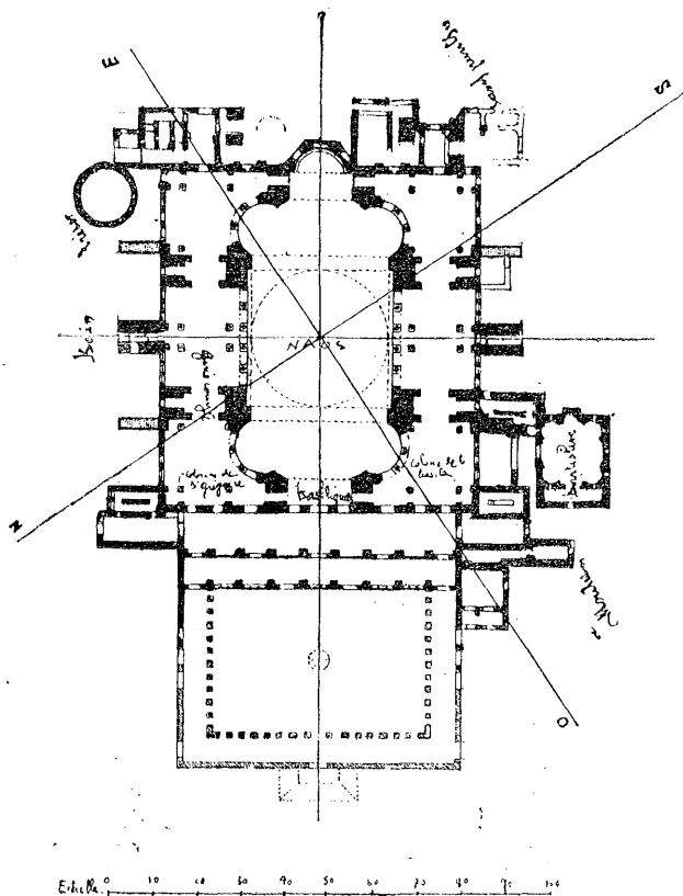
Планъ собора св. Софiя.
